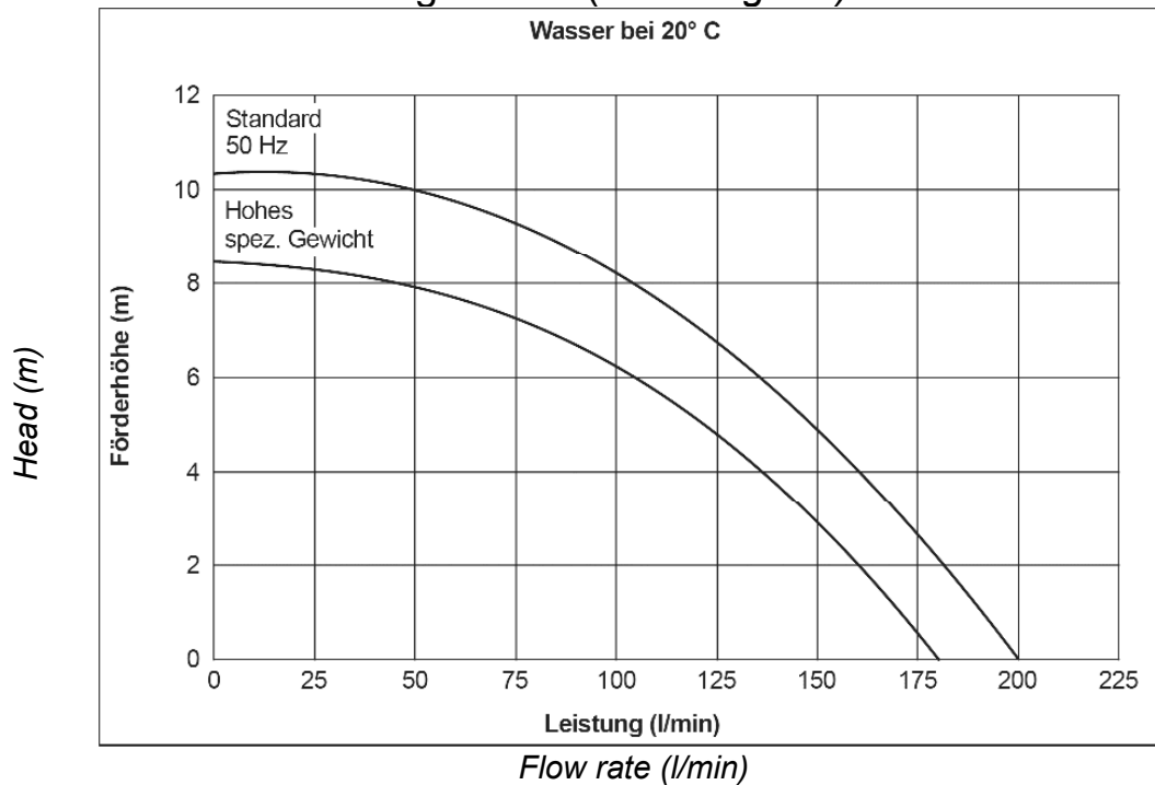
Leistungskurve* (load diagram)* 50Hz
