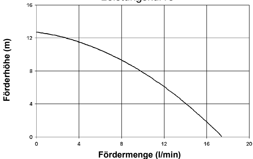
Leistungskurve*
