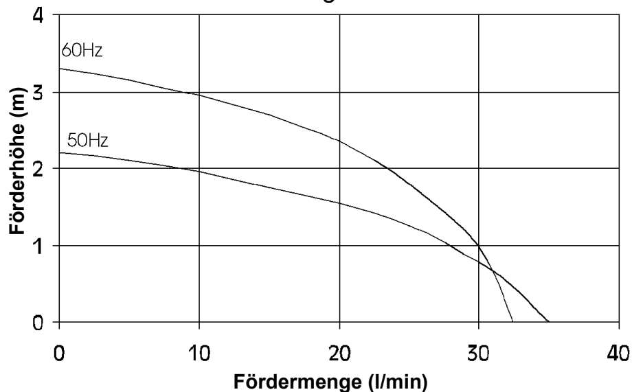
Leistungskurve*
