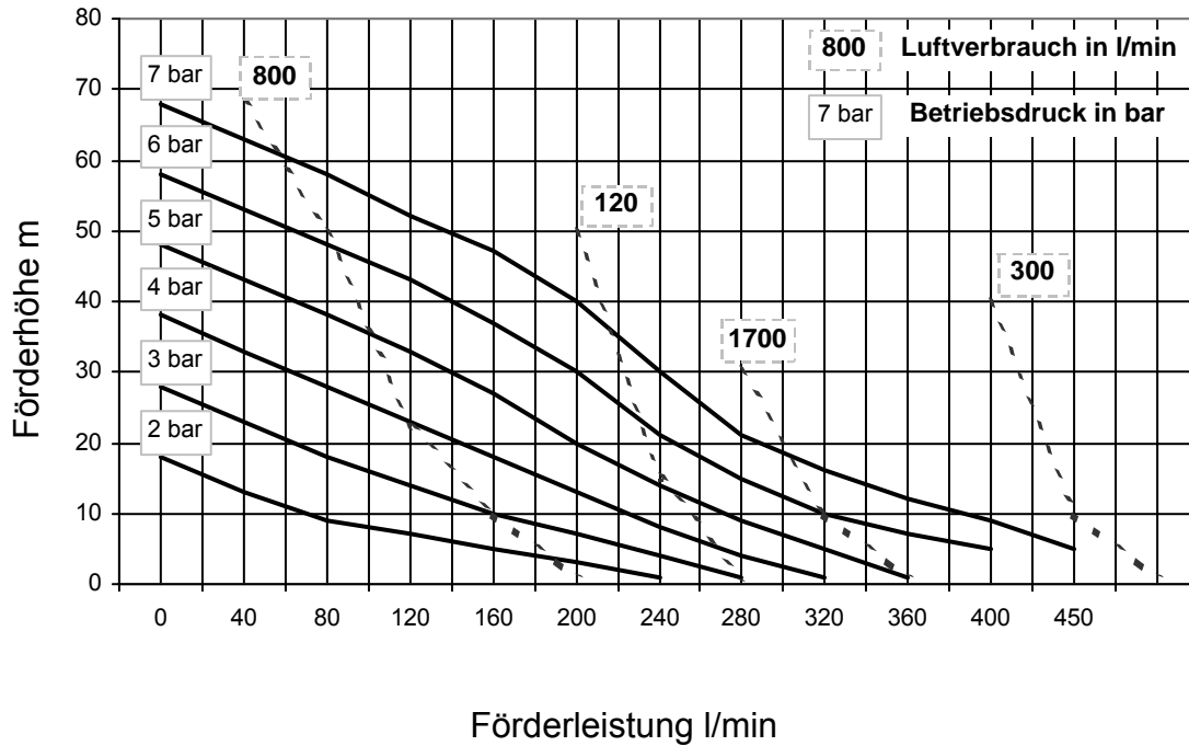
Leistungsdiagramm DMP 500
