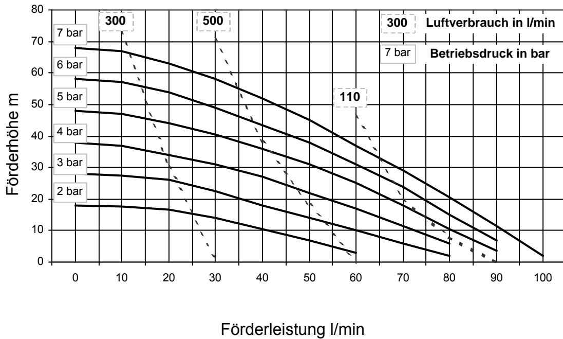
Leistungsdiagramm DMP 81 AL
