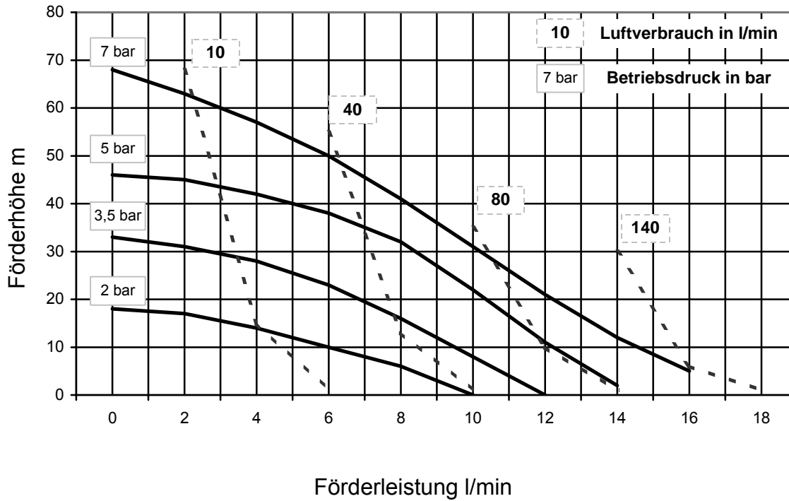
Leistungsdiagramm DMP 15
