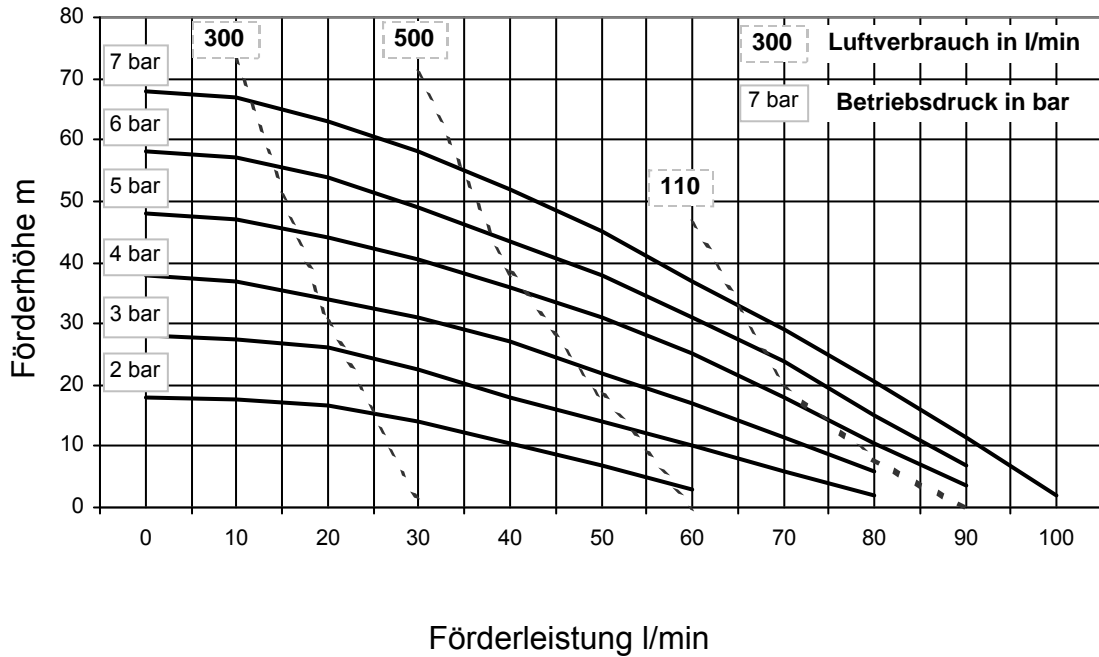
Leistungsdiagramm DMP 81 AL
